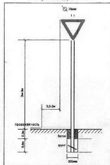
Схема установки дорожного знака
