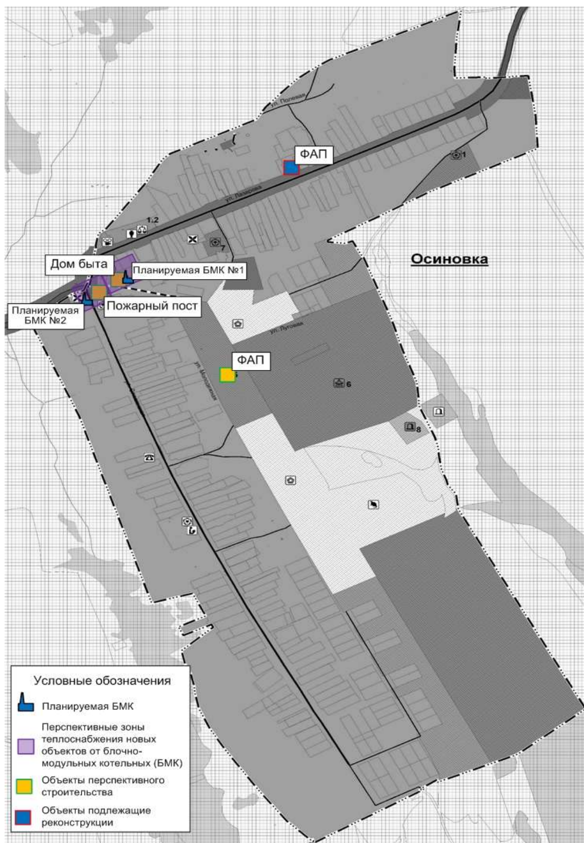
Рис. № 14 - Перспективные зоны теплоснабжения блочно-модульных источников тепловой энергии, планируемых к размещению на территории, села Осиновка
