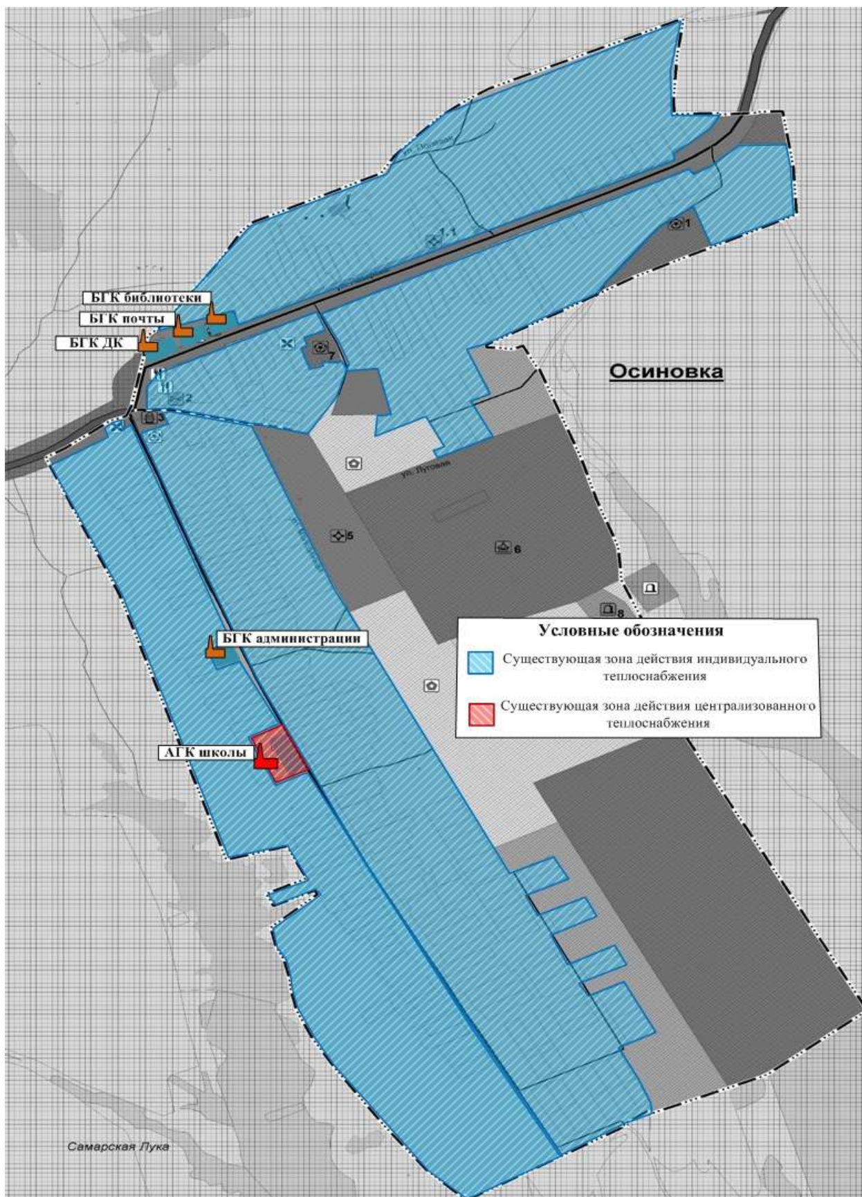
Рис. № 6 - Зоны действия АГК и индивидуальных источников тепловой энергии на территории села Осиновка
